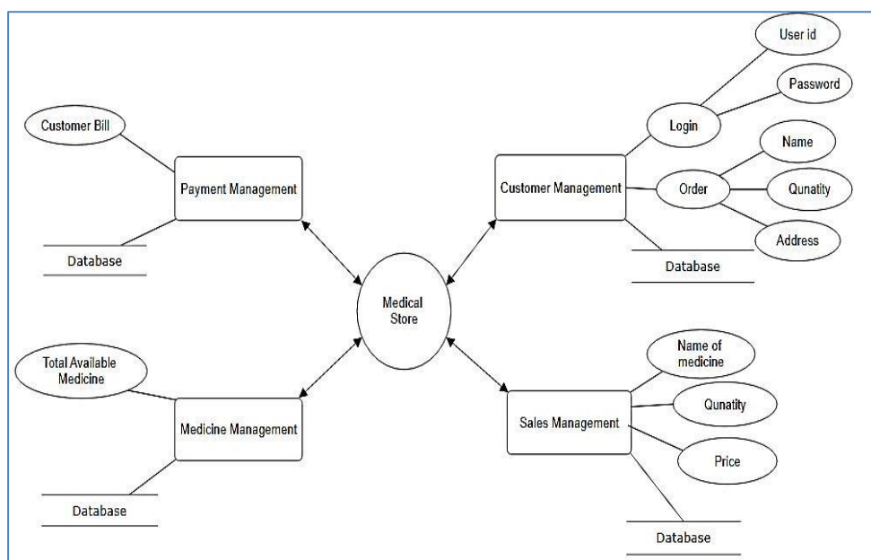
Fig. 1: DFD Level-2
