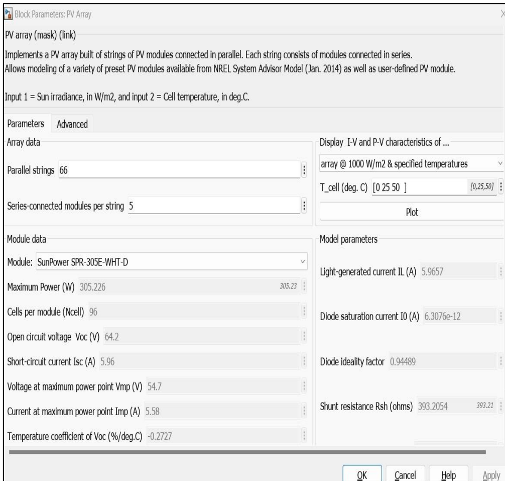
Fig. 5: PV array parameters
